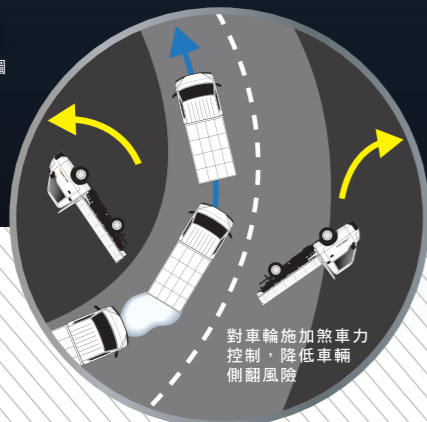
ARP主動式防止傾覆系統
