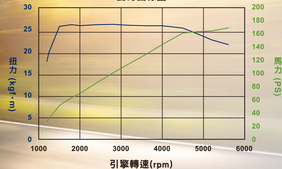
動力曲線圖
