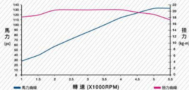
引擎性能曲線圖
