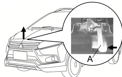
A - 控制桿
